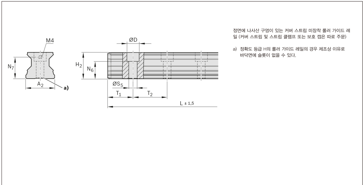
치수 (mm)
